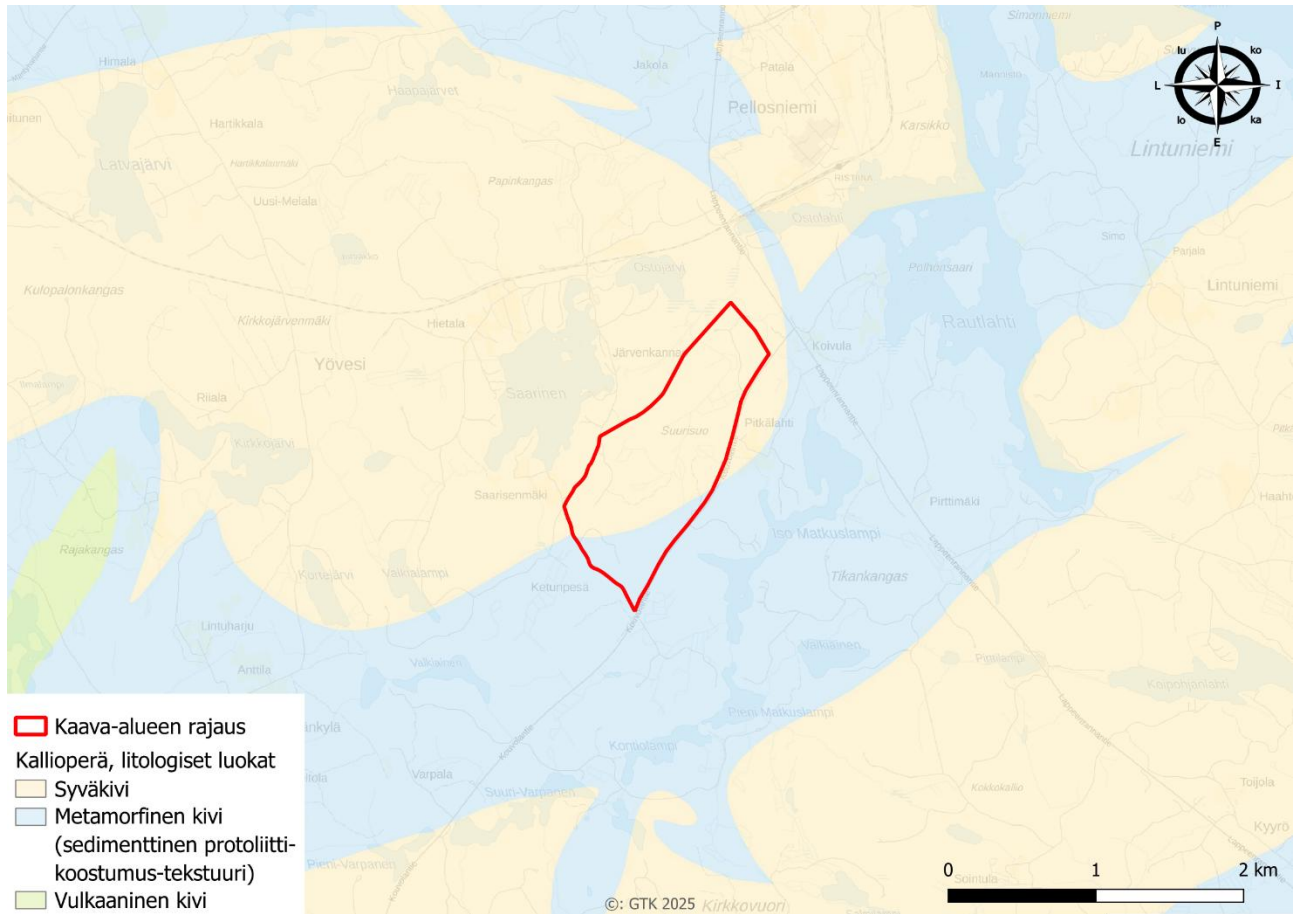
Kuva 14. Kallioperä.
